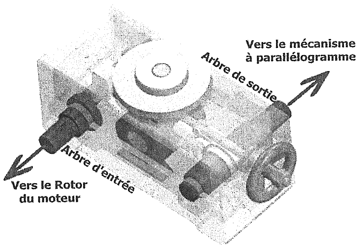
Figure 4 : Excitateur mécanique à amplitude réglable
