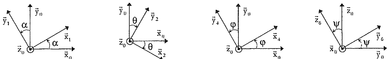
Figure B.2 : Représentation plane des rotations
