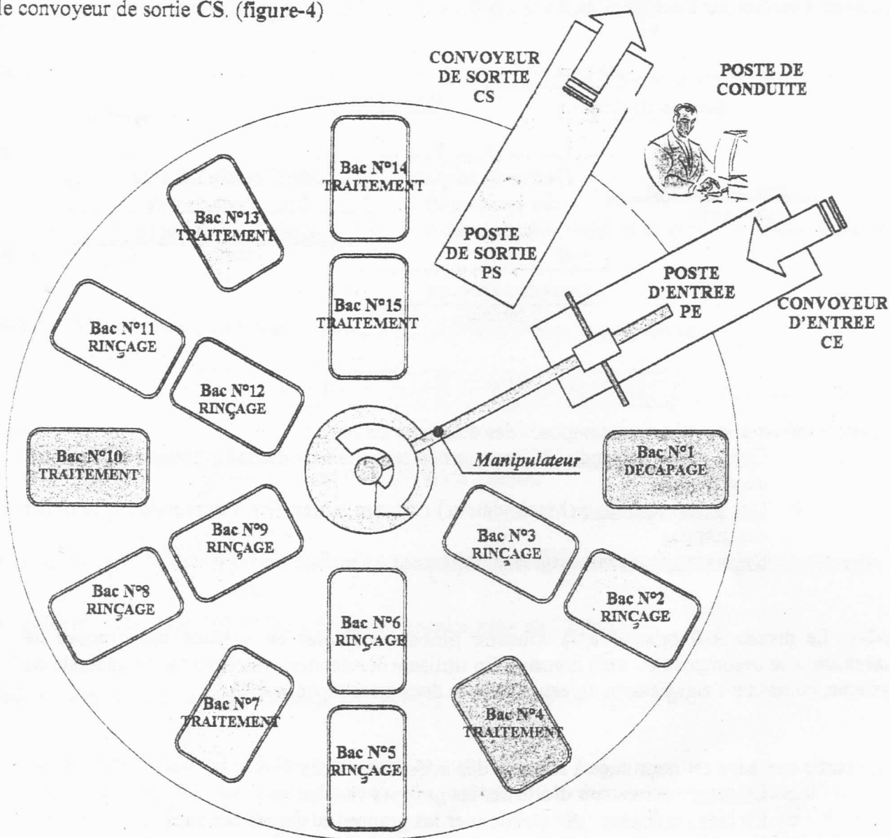
Figure-4 : Disposition générale de l'unité de traitement
