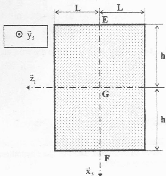
Figure-B.3 : Plaque rectangulaire homogène dans le plan (E, \vec{x}_1, \vec{z}_1) .
