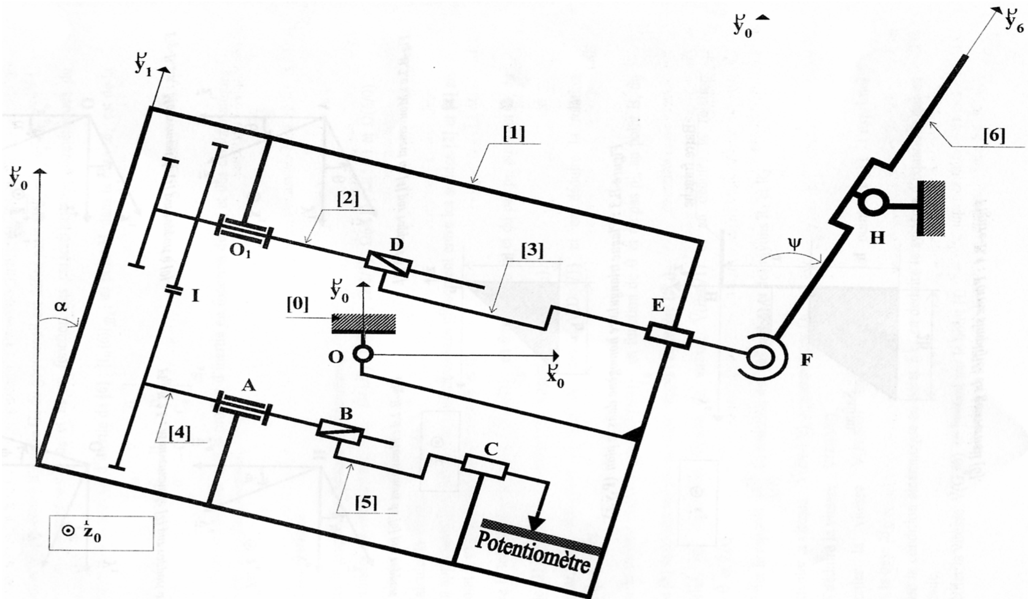
Figure-B.1 : Schéma cinématique du mécanisme.
