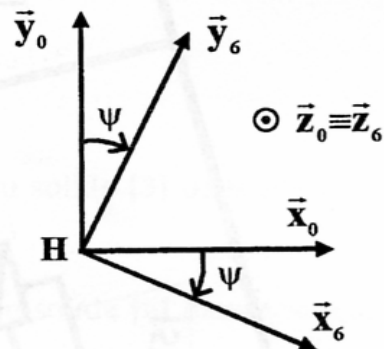
Fig-B.2.d : Mouvement de [6] par rapport à [0].
