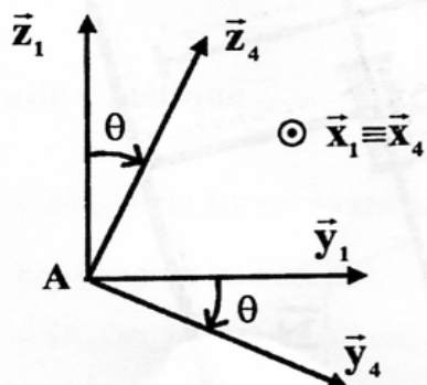
Fig-B.2.c : Mouvement de [4] par rapport à [1].
