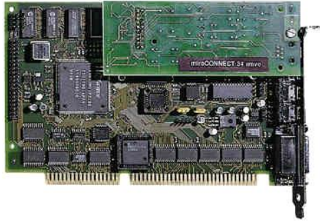
Carte fax modem
