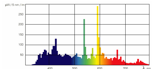
Spectre d'une lampe à iodure métallique (Mazda)
