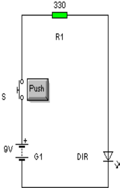
دارة البث
