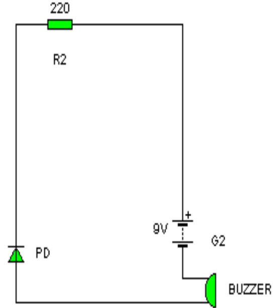
دارة المتقبّل
